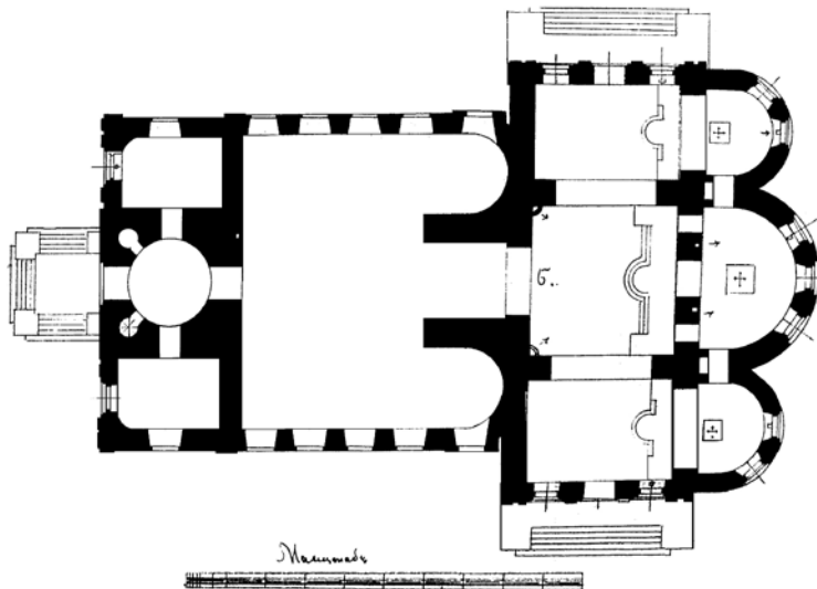
Рисунок 4 – Реконструкция плана церкви на сер. XIX в.
