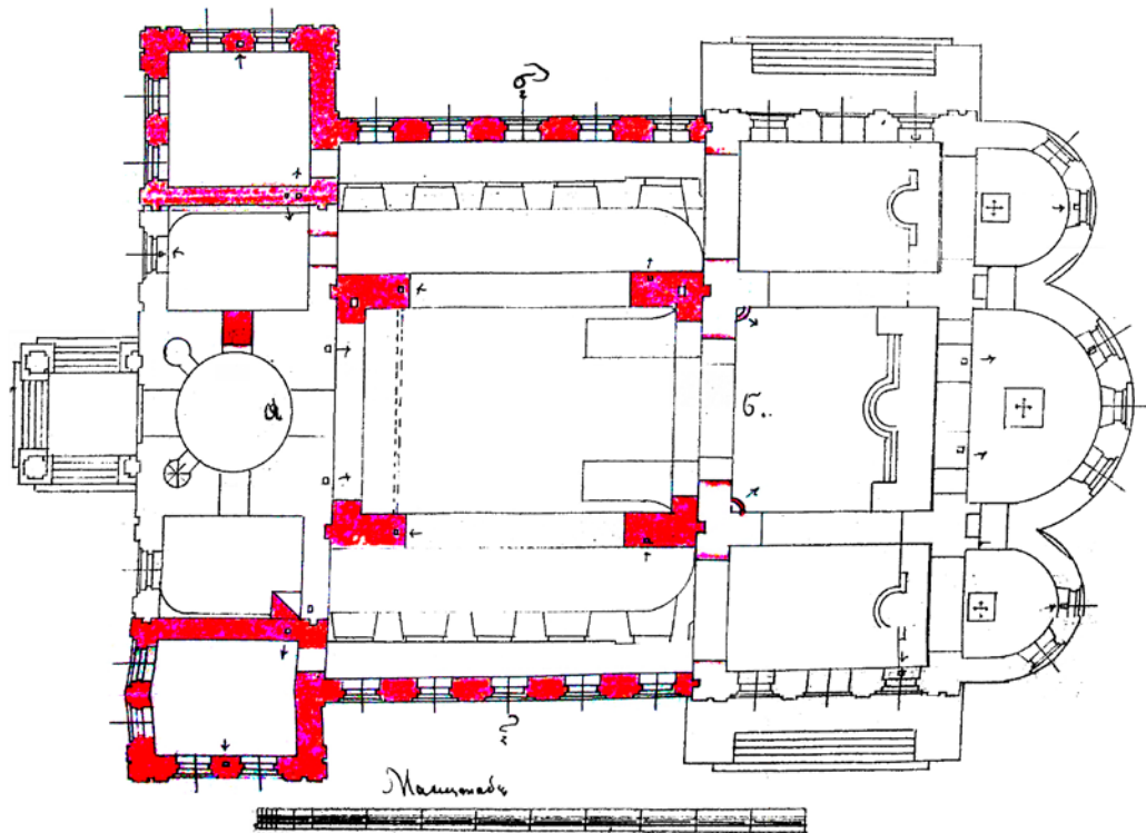
Рисунок 5 – План переустройства храма в селе Сада. ГАКО ф.583, оп.528, ед.хр.232. Чертеж И.А. Чарушина, 1907 г.
