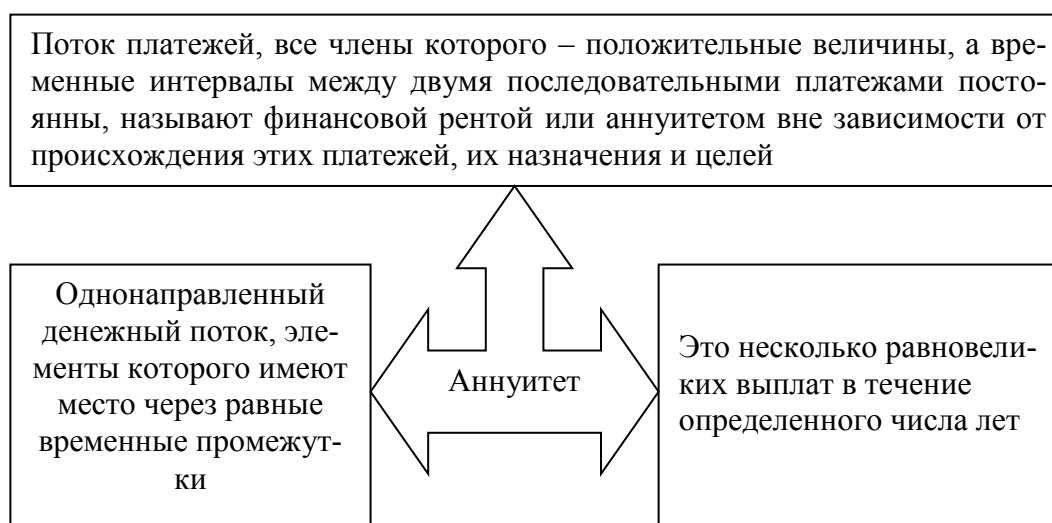
Рис.2. Определения аннуитета
