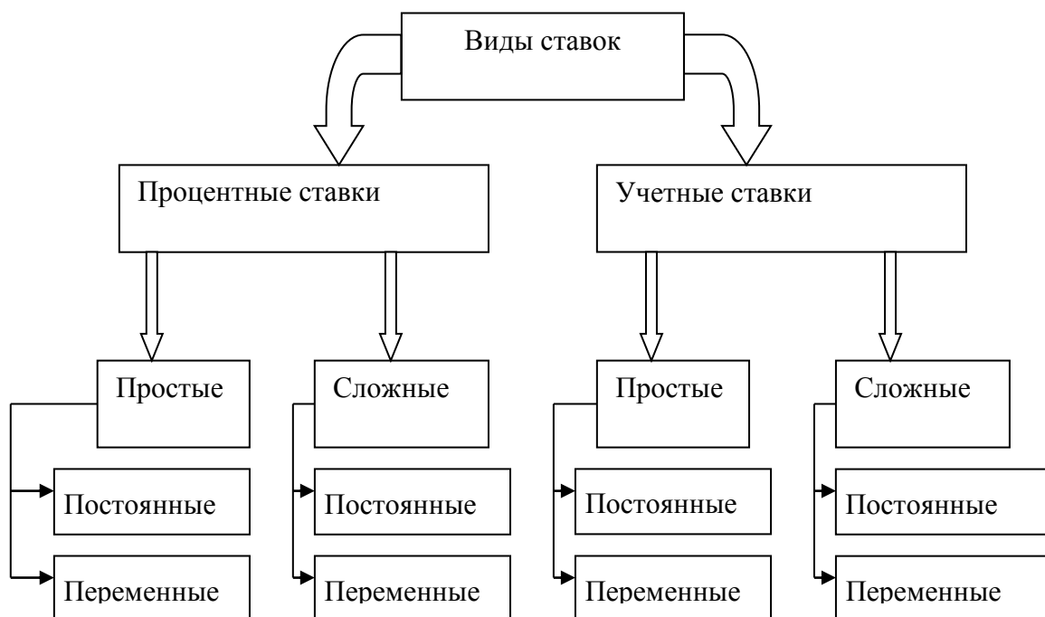
Рис.1. Классификация ставок
