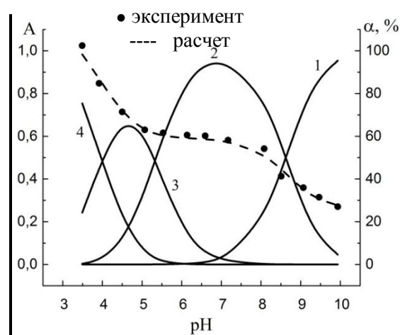
Рис. 2. Зависимость оптической плотности (A) растворов Pd(II)–HTФ от кислотности среды и диаграмма распределения комплексов ( \alpha , %) в растворе.
