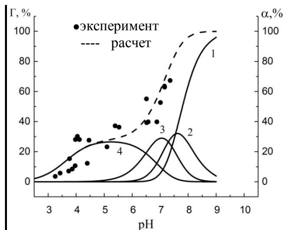
Рис.1. Зависимость степени сорбции Pd(II) на HTФ- \gamma -AlO(OH) от кислотности среды (Г, %) и диаграмма распределения комплексов ( \alpha , %) на поверхности.
