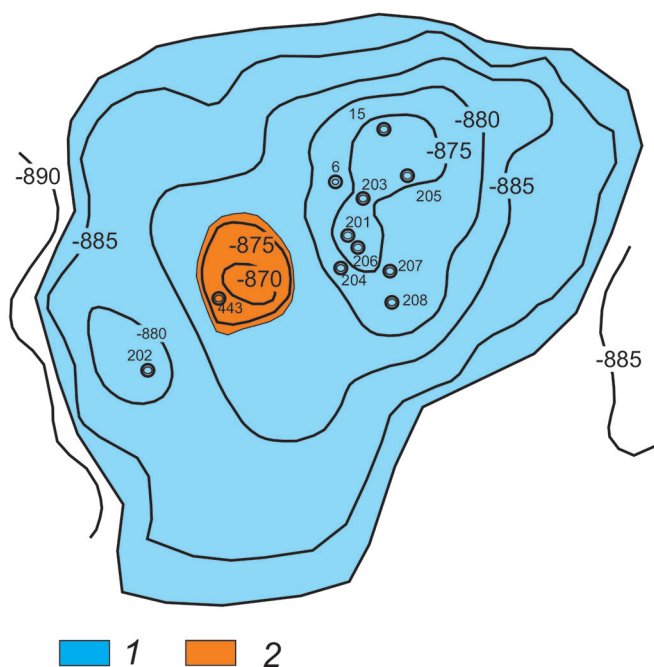
Рис. 1. Несовпадение предполагаемой и фактической площади нефтегазоносности: 1 — предполагаемая зона нефтегазоносности; 2 — фактическая зона нефтегазоносности
