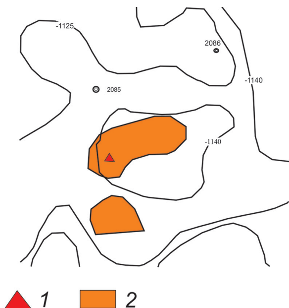
Рис. 3. Применение технологии АНЧАР для выявления пропущенных залежей на примере Староягинской структуры: 1 – рекомендованное расположение скважин; 2 – внешний контур нефтегазоносности
