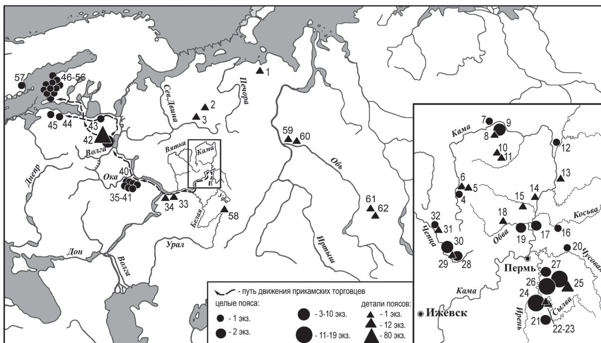
Рис. 2. Схема распространения поясов неволинского типа:
