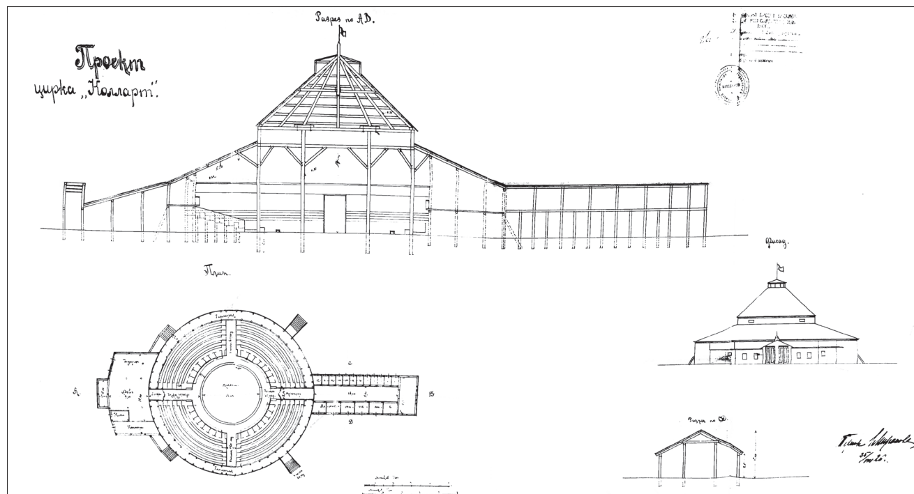
Рис. 1. Проект цирка «Колларт». Чертеж 1926 г., из фондов ЦГА УР
