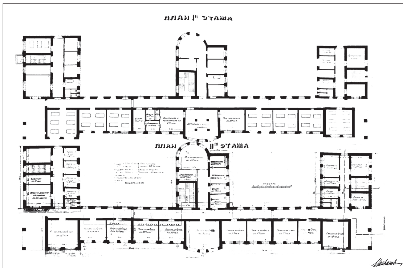
Рис. 2. Проект Областной больницы в Ижевске. Чертеж 1928 г., из фондов ЦГА УР
