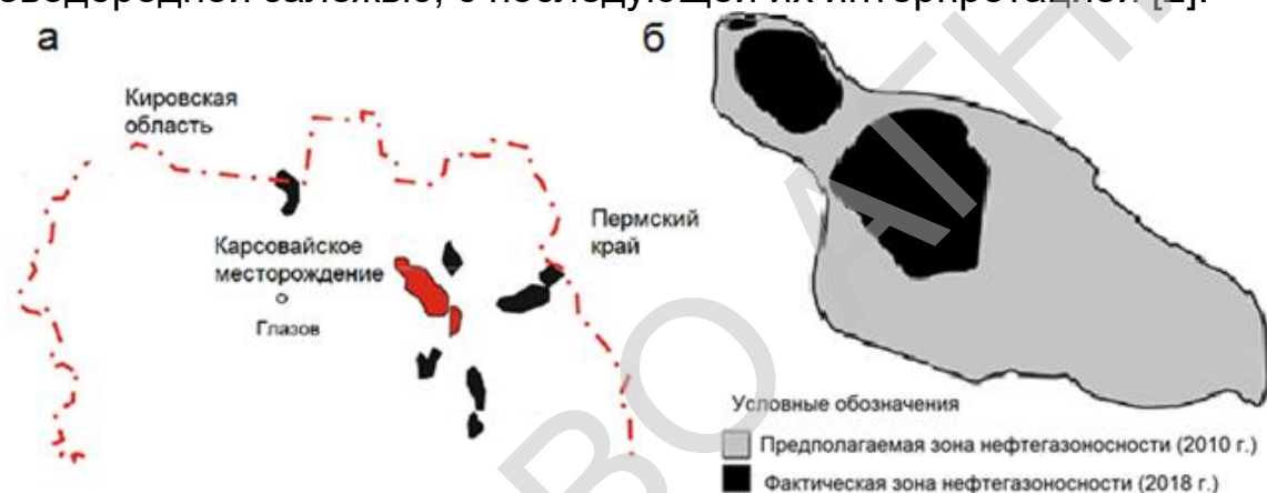
Рисунок 1 - Схема расположения (а) и схема с выделенными зонами предполагаемой и фактической нефтегазоносности (б) Карсовайского месторождения
