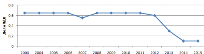
Рисунок 1 – Динамика среднегодовых концентраций содержания загрязняющих веществ в атмосферном воздухе г. Ижевска за 2003-2015 гг.
