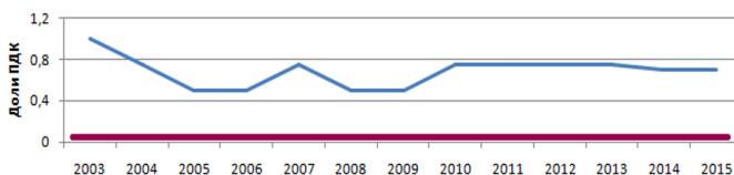
Рисунок 2 – Динамика среднегодовых концентраций содержания \text{NO}_x в атмосферном воздухе г. Ижевска за 2003-2015 гг.
