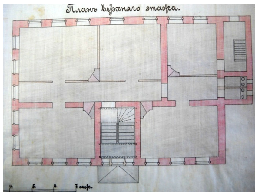
Рис. 3. План на постройку каменного двухэтажного корпуса для детского приюта в Ижевском заводе Вятской губ. Сарапульского уезда. 1899 г. План верхнего этажа. Проект не утвержден и не реализован Источник: [16].
