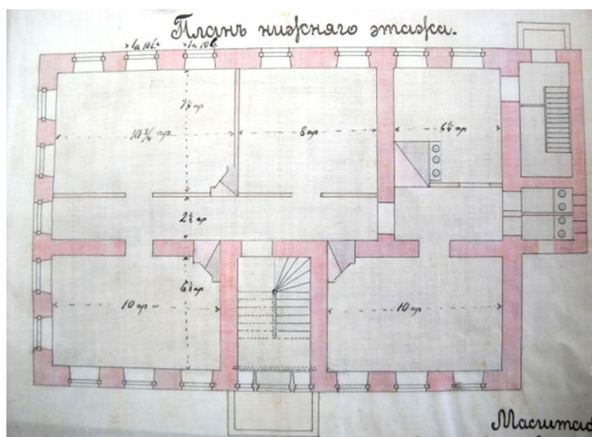
Рис. 2. План на постройку каменного двухэтажного корпуса для детского приюта в Ижевском заводе Вятской губ. Сарапульского уезда. 1899 г. План нижнего этажа. Проект не утвержден и не реализован Источник: [16].
