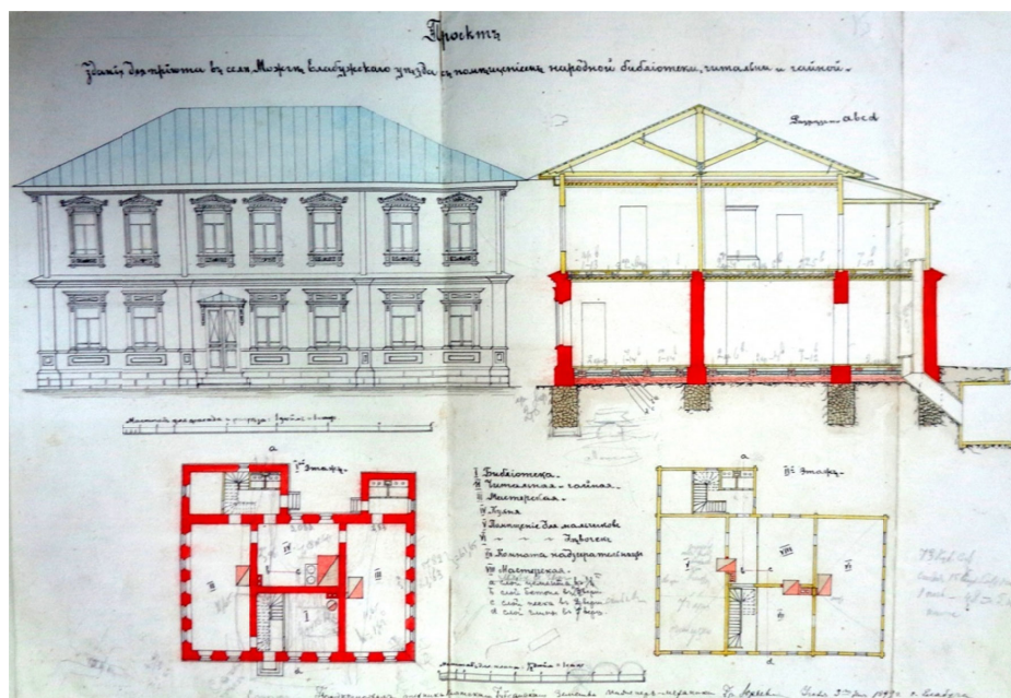
Рис. 6. Проект здания для детского приюта в с. Можга Елабужского уезда с помещением народной библиотеки, читальни и чайной Источник: [16].
