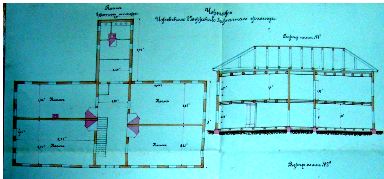
Рисунок 2. Чертеж Ижевского 2 мужского заречного училища. ГАКО, ф.205, оп.4, ед.хр.3220. Об открытии в Ижевской заречной волости высшего начального училища. 1914 г.
