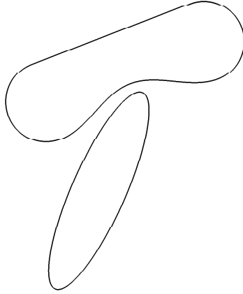
Рис. 4: Множества, не являющиеся отделимыми.
