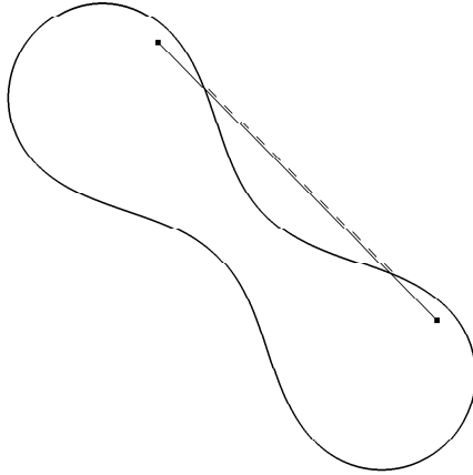
Рис. 2: Множество, не являющееся выпуклым.
