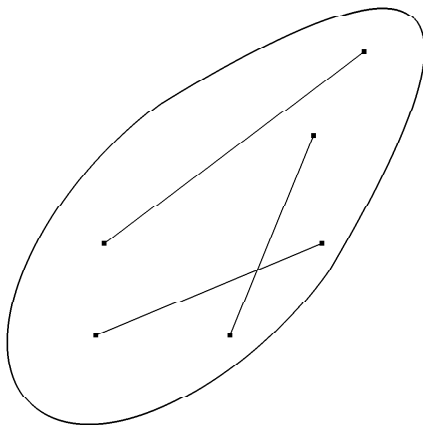
Рис. 1: Выпуклое множество.
