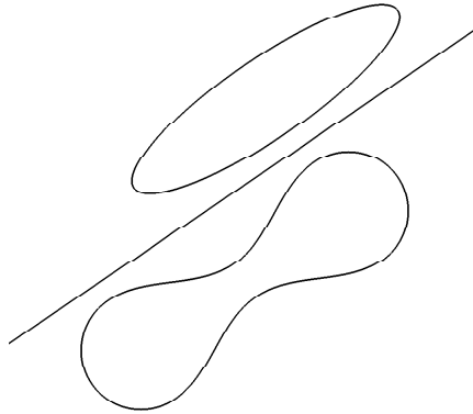
Рис. 3: Отделимые множества.
