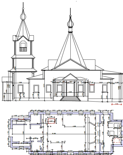
Предварительные кроки по обмерам 2018 г.: план, южный фасад. Архитекторы Д. Н. Ральников, Т. Шанина
