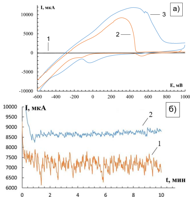
Рисунок 1. а) Циклическая вольтамперограмма СУ электрода(1), СУ/Pd электрода(2), СУ/хитозан/Pd электрода(3). Электролит 0,1М H 2 SO 4 . Скорость развертки потенциала 20мВ/с.б) Хроноамперограмма СУ/Pdэлектрода (1) и СУ/хитозан/Pd электрода (2). Потенциал -0,6 В.
