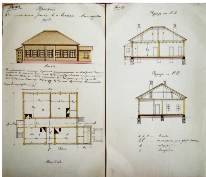
Проект школьного здания в с. Селтах Малмыжского уезда. 1902 г. Источник: ЦГАКО
