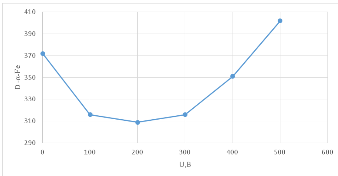
Рис. 1. Зависимость ОКР от подаваемого смещения напряжения
