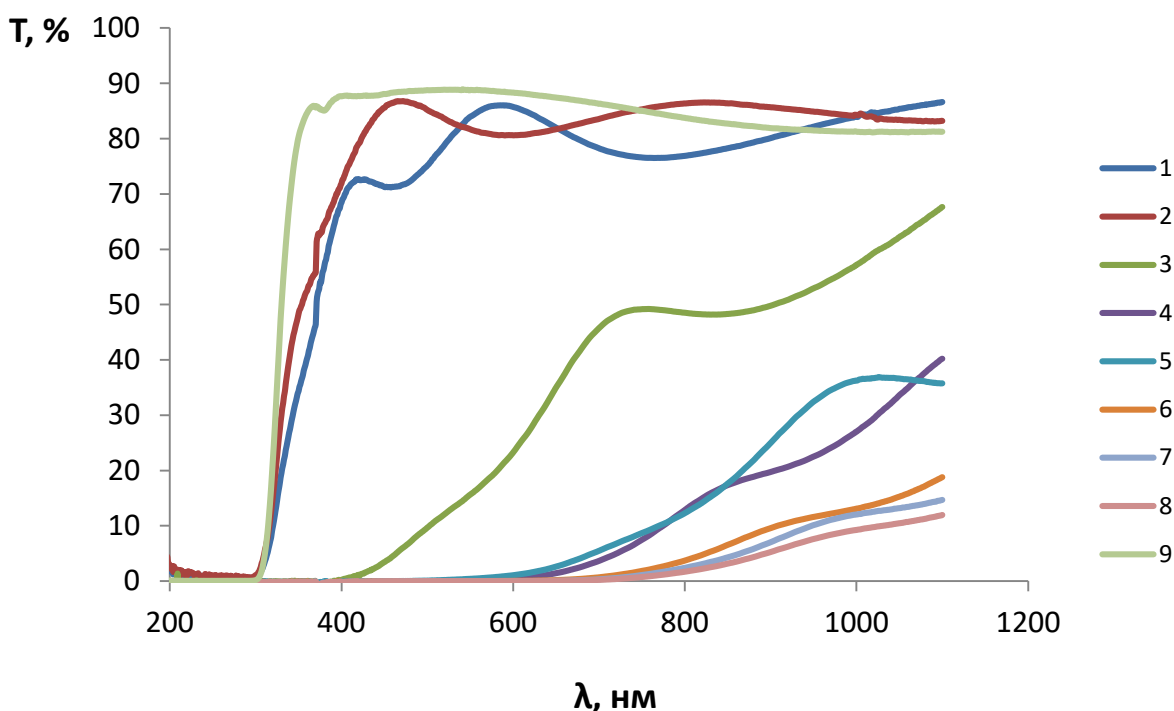
Рисунок 1. Спектры пропускания мультислойных структур PbS-Al 2 O 3 с толщиной слоев Al 2 O 3 и толщиной слоев PbS 6 Å (1), 8.2 Å (2), 16.4 Å (3), 24.6 Å (4), 32.8 Å (5), 49.6 Å (6), 65.5 Å (7), 131.2 Å (8) Å, подложки (9).
