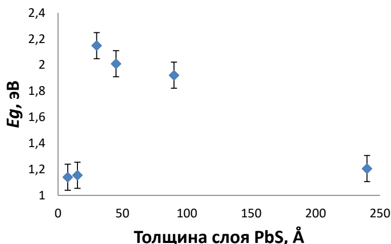
Рисунок 1. Зависимость ширины запрещенной зоны нанокompозитных систем PbS-SiO 2 от толщины слоев сульфида свинца.
