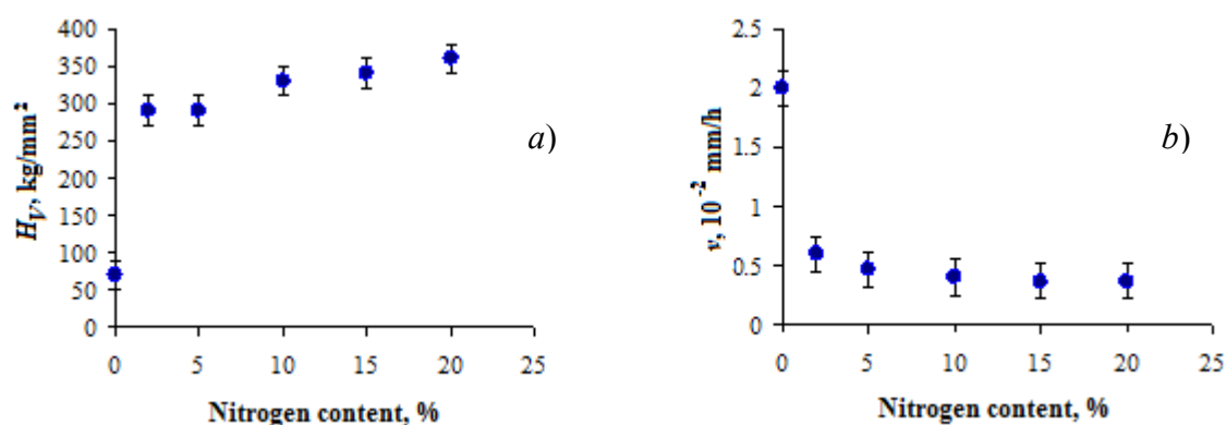
Рис. 4. Изменение микротвёрдости образцов с напылёнными плёнками нитрида титана с последующей ионно-лучевой обработкой (а) и зависимость скорости истирания (b) образцов с напылёнными плёнками нитрида титана от процентного содержания азота в рабочей смеси
