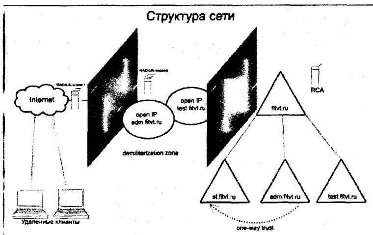
Схема сети представлена на рис. 2.
