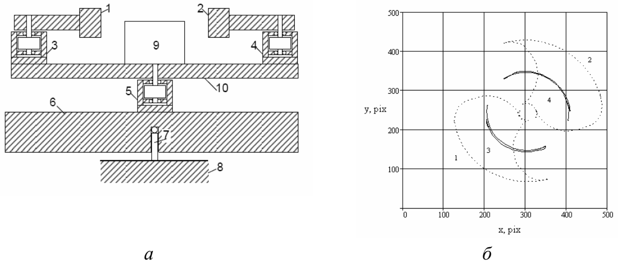
Рис. 5. Кинематическая схема мехатронной модели (а) и результат идентификации траекторий подвижных частей модели (б)
