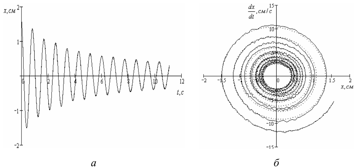
Рис. 3. Свободные демпфированные колебания: а – зависимость координаты от времени, б – фазовая траектория; сплошная линия – эксперимент, пунктир – результат аппроксимации квадратичным трением
