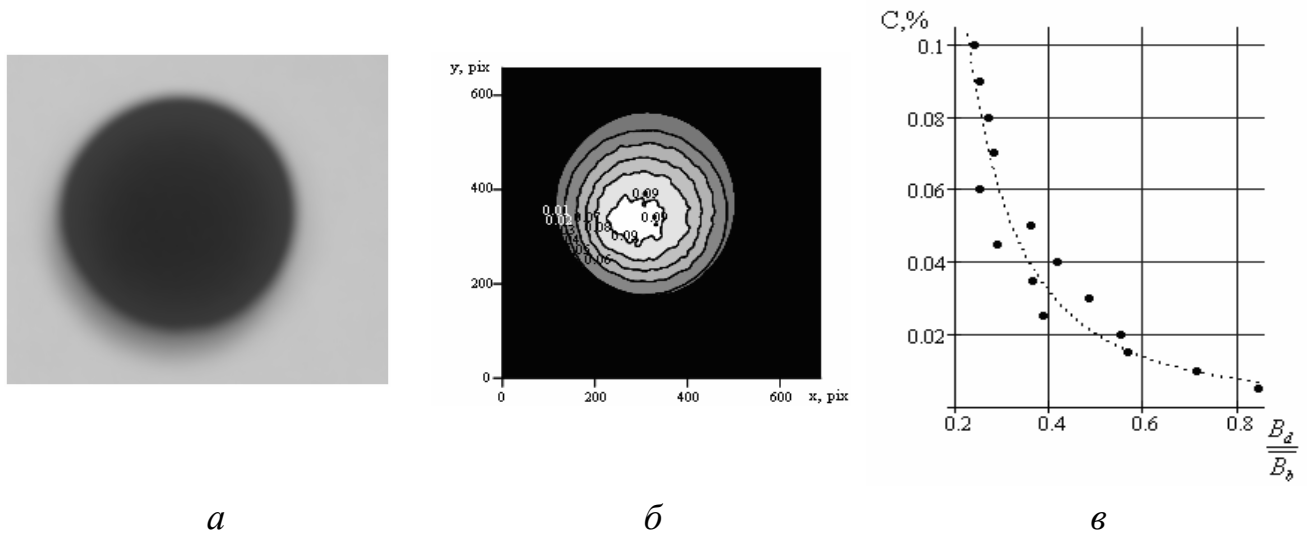
Рис. 6. Восстановление поля концентрации для красного тканевого красителя: а – диффузионное пятно, б – поле концентрации, в – калибровочная зависимость
