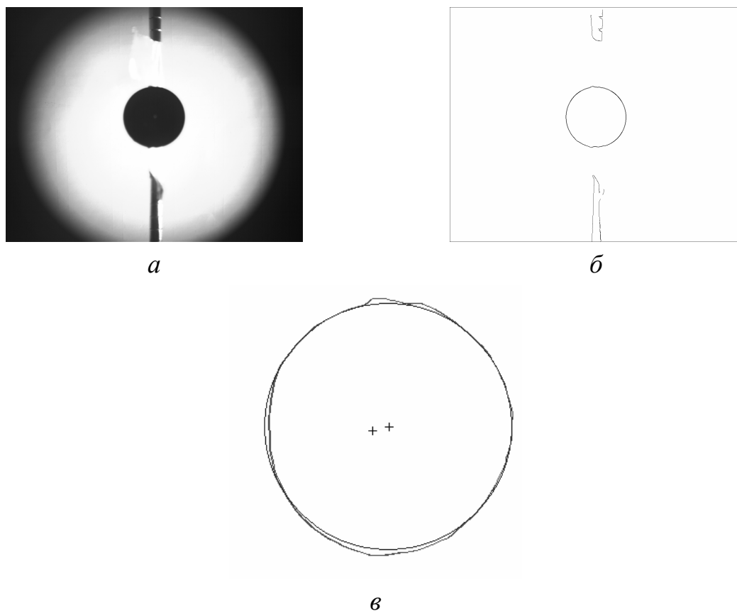
Рис. 2. Изображение маятника (а), выделенные контуры (б), определение центра метки (в)
