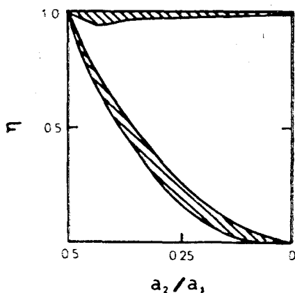
Рис. 2. Области существования эллипсоидов с наклонным вращением.
