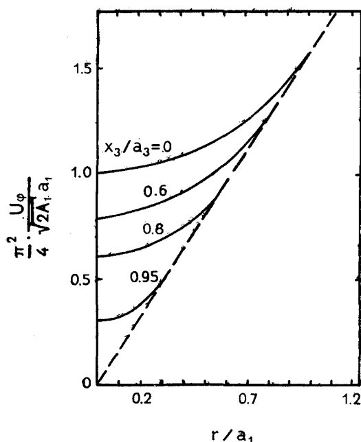
Рис. 5. Кривые вращения при разных \frac{x_3}{a_3} для модели с f_{rz}^{(2)} = 0 . Все кривые имеют одну касательную, что связано с твердотельным характером осредненного вращения поверхности модели. Причина неисчезновения вращения на оси x_3 объяснена в тексте.
