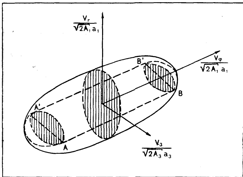
Рис. 4. Объемное изображение фигуры, показанной на рис. 3. По краям ее заштрихованы линзовидные сечения, посредине — окружность с радиусом \sqrt{\beta - \alpha} .
