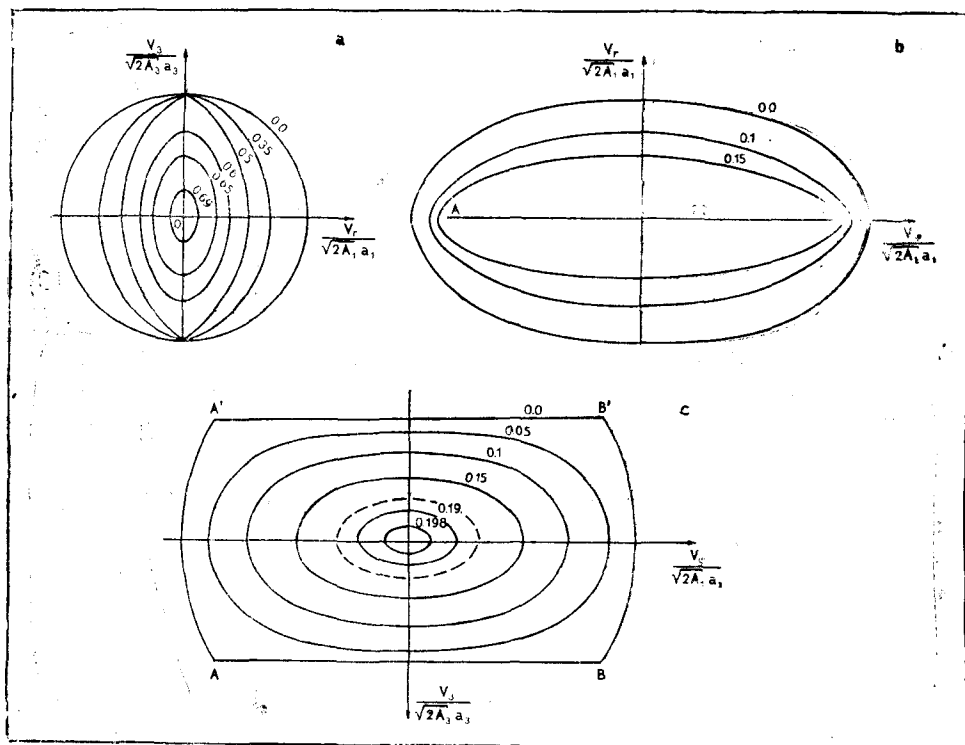
Рис. 3. Сечения фигуры, поверхность которой представляет собой область существования модели в пространстве скоростей. Для расчетов взято \alpha = 0.3 и \beta = 0.5 . а) Плоскостями, параллельными осям 0v_z v_r ; цифрами обозначены контуры сечений при разных значениях \frac{v_r^2}{2A_1 a_1^2} . Внешний контур—окружность радиусом \sqrt{\beta-\alpha} ; контур \frac{v_r^2}{2A_1 a_1^2} = 1 - \beta представляет линзу с острыми краями (где производная терпит разрыв). б) Плоскостями, параллельными осям 0v_r v_z ; цифрами обозначены значения \frac{v_z^2}{2A_3 a_3^2} . Контур-семейство софокусных эллипсов, межфокусное расстояние AB равно 2\sqrt{1-\beta} . в) То же самое плоскостями, параллельными осям 0v_z v_r ; цифрами даны значения \frac{v_r^2}{2A_1 a_1^2} . Внешний контур состоит из двух отрезков длиной 2\sqrt{1-\beta} , соединенных дугами окружности с радиусом \sqrt{1-\alpha} .
