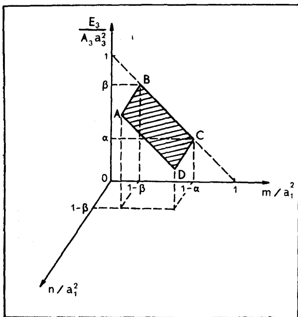
Рис. 2. Заштрихована область, занимаемая моделью в пространстве интегралов движения отдельной частицы.
