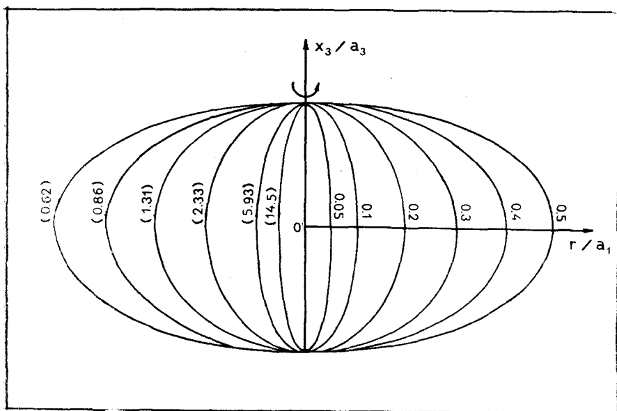
Рис. 6. Сечения поверхностей равного среднего эксцентриситета экваториальных разрезов орбит частиц; цифрами без скобок даны значения квадрата среднего эксцентриситета. Цифры в скобках — значения средней угловой скорости вращения центроидов, нормированной на фактор \sqrt{\pi G \rho} . Указанное относится только к модели с вращением частиц в одну сторону. Для вычислений взята модель сжатого сфероида с a_3/a_1 = 0.5 .
