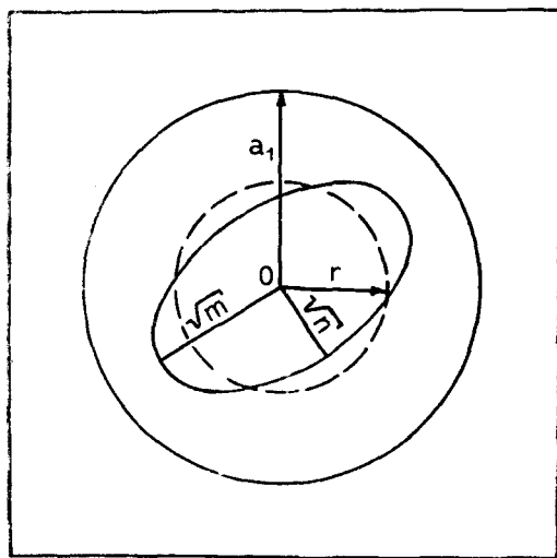
Рис. 1. Сечение эллиптического цилиндра, поверхность которого покрывает частица при движении, экваториальной плоскостью модели.
