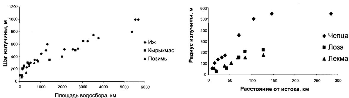
Рис. 3. Изменение радиуса и шага излучин на отдельных реках Удмуртии
