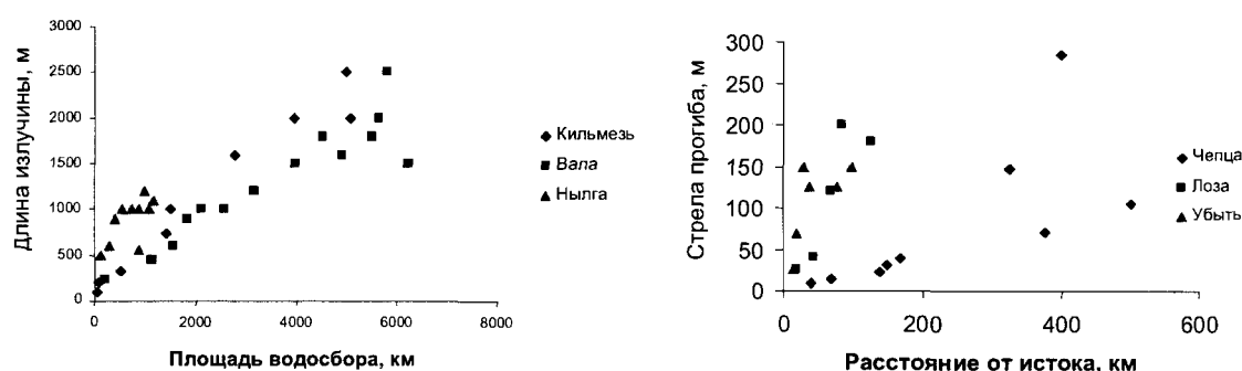
Рис. 4. Изменение длины и стрелы прогиба излучин на отдельных реках Удмуртии
