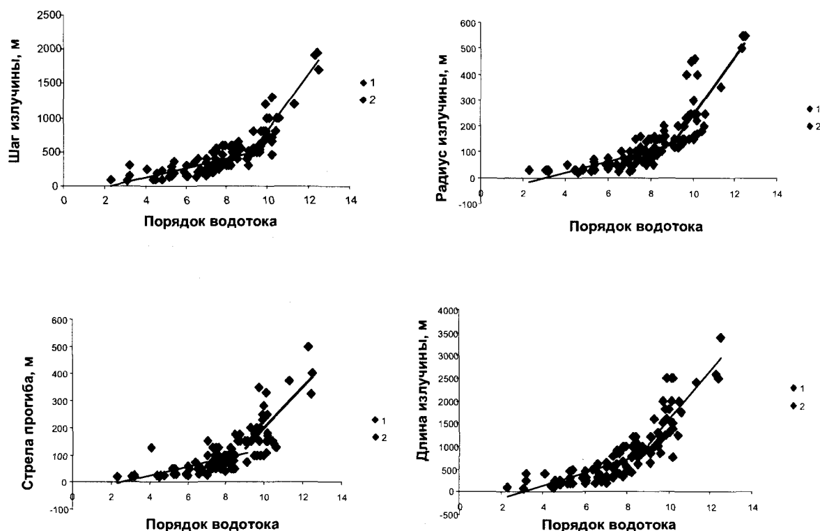
Рис. 5. Изменение параметров свободных излучин на реках различных порядков: 1 – реки до 9-го порядка; 2 – реки с порядком 9 и выше
