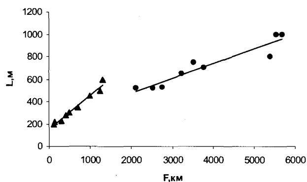
Рис. 6. Зависимость характерных значений шага свободных излучин ( L_m ) р. Ижа от площади водосбора ( F, \text{км}^2 ): 1 – для рек до 9-го порядка; 2 – для рек с порядком 9 и выше
