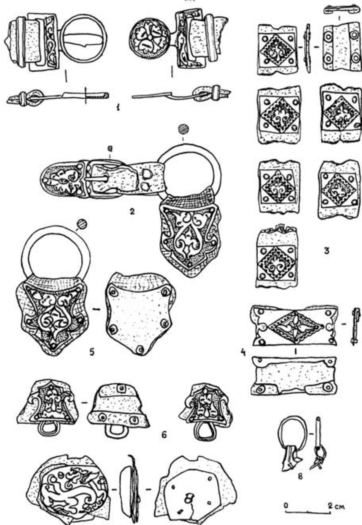
Рис.61. Детали серебряного поясного набора из погребения 4 мавзолея, раскопанного в 1913 г. на Увекском городище (общий музейный № СМК ДЗ-23).
