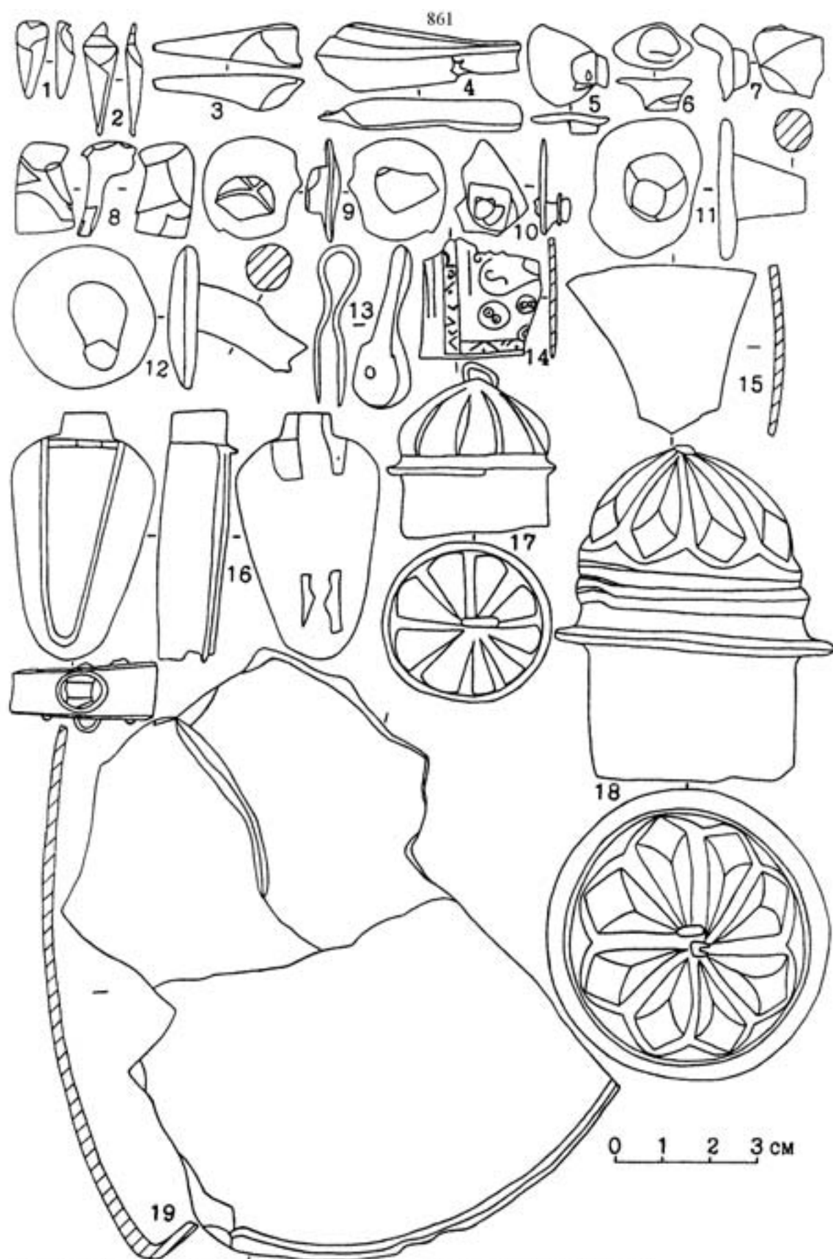
Рис. 75. Бронзовые сосуды и их части. Увекское городище. 1-12 - заклепки, 13 - ушко, 14-15 - стенки, 16 - флакон, 17-18 - крышки, 19 - днище. 1-11, 14, 16 - СМК №/№ 1223; 1229; НВСП 18037 (СУАК 1776); 1220; 1222/6; 1228 (ст. № 1851); НВСП 29781 (СУАК 2360/4; АО 288). 12-13, 15, 17-19 - НМРТ №/№ 5365-32; 5365-20 (АА 40-16); 5365-7 (ст. № 20689); 5365-30, ОАИ-20, ст. № 18439.
