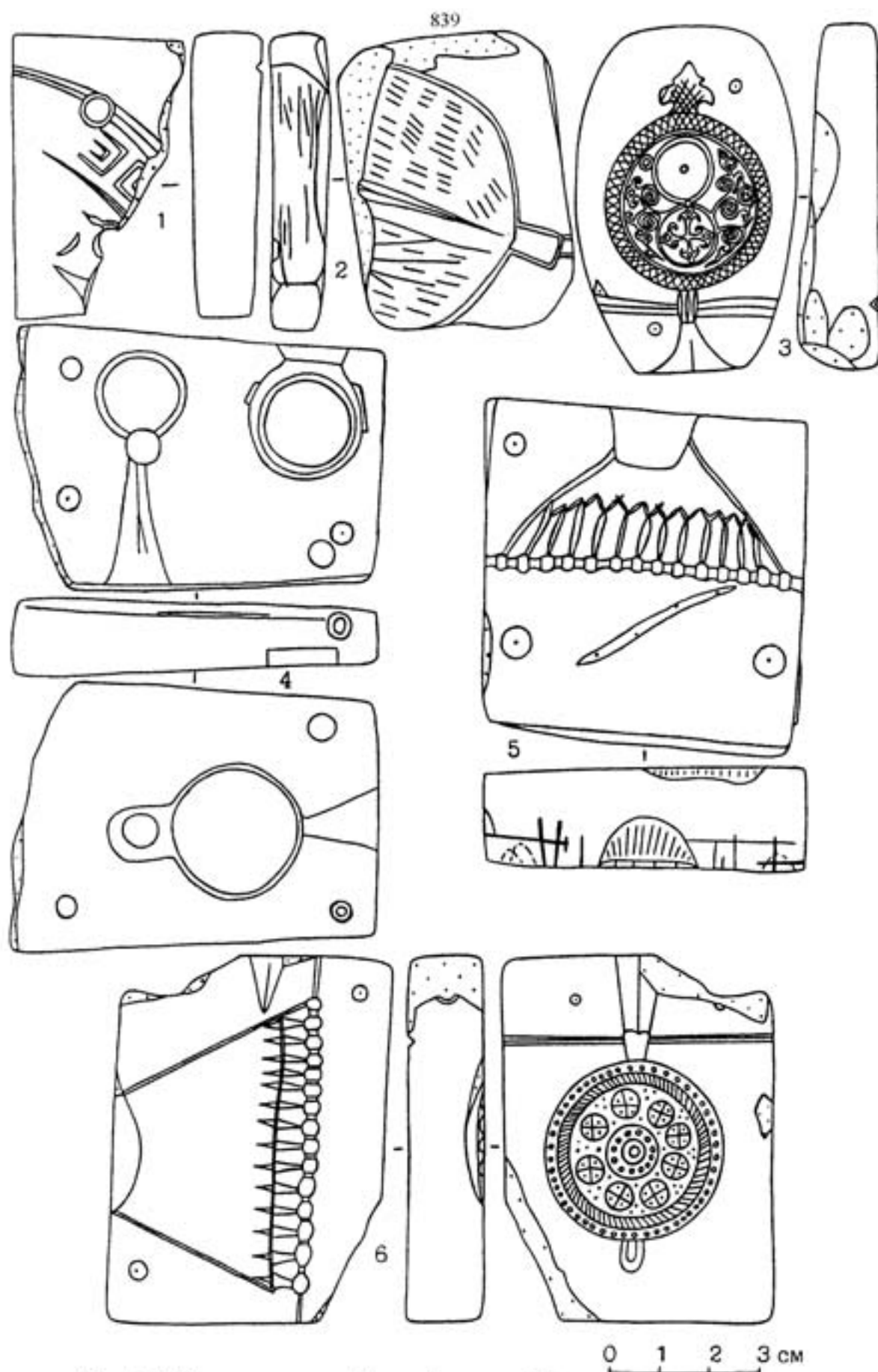
Рис.59. Каменные литейные формы с Увекского городища.
