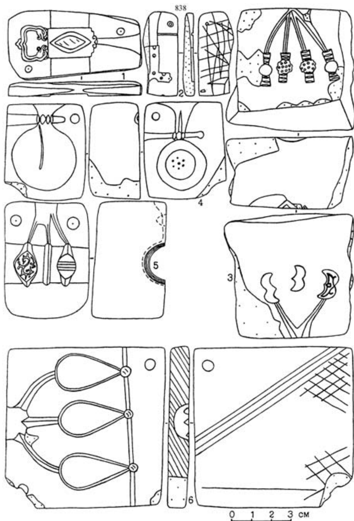
Рис.58. Бронзовая (1) и каменные (2-6) литейные формы с Увекского городища.
