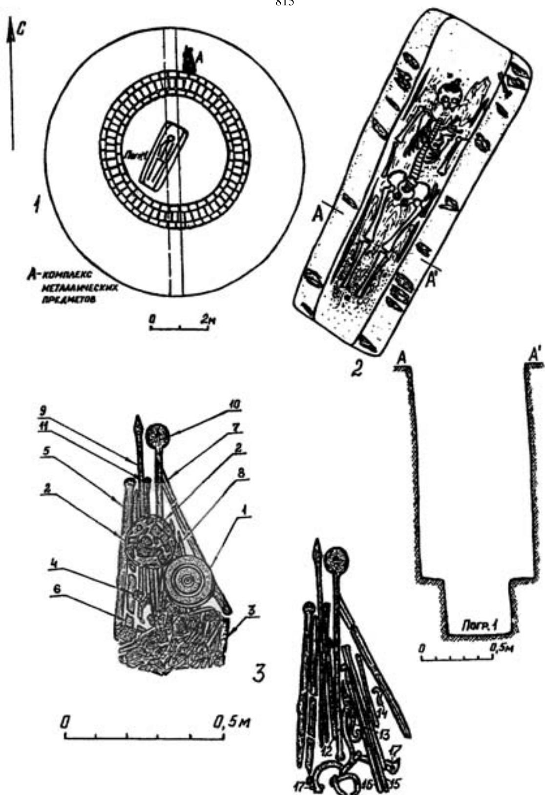
Рис.38. Комплекс кузнечного инструментария в насыпи кургана 4 группы Маляевка VI (по: Мыськов Е.П. Погребальные сооружения с кирпичными оградами могильника Маляевка VI у северо-западного пригорода Царевского городища // НАВ.- Волгоград: Изд-во Волгоградского государственного университета, 2003.- Вып.6.- С.232, рис.6).
