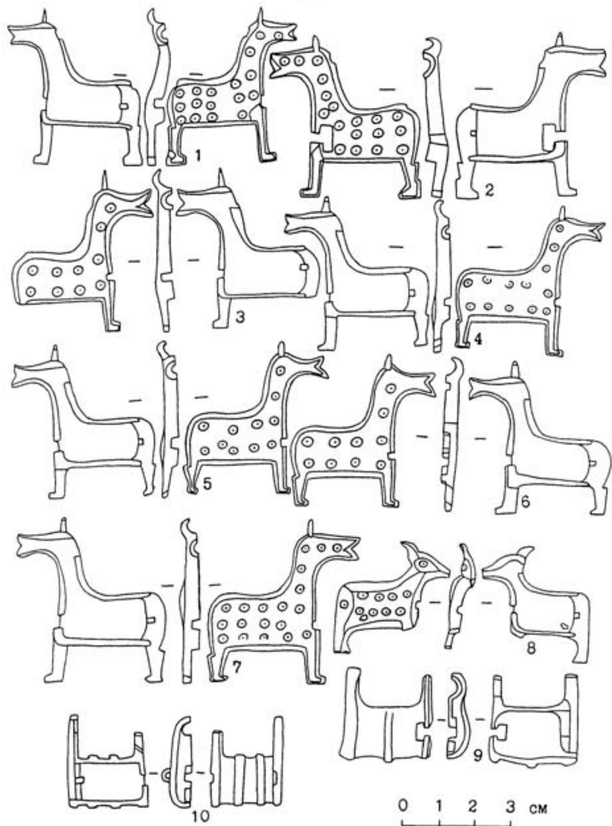
Рис. 78. Половинки бронзовых замочков с Увекского городища. 1-3, 9-10 - СОМК №/№ АО 1244/1-3, НВСП 29779 (АО 288/4), 1245/4. 4-8 - НМРТ № 5365-9.
