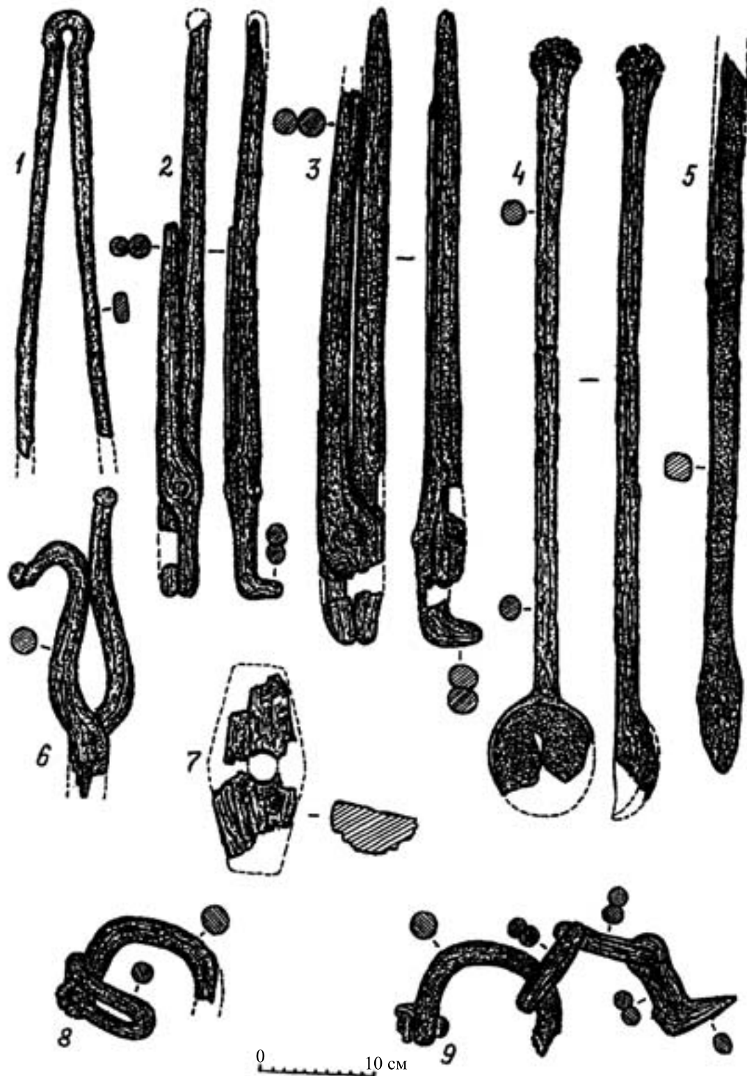
Рис.39. Кузнечные инструменты и другие изделия из комплекса в насыпи кургана 4 группы Маляевка VI (по: Мыськов Е.П. Погребальные сооружения с кирпичными оградами могильника Маляевка VI у северо-западного пригорода Царевского городища // НАВ.- Волгоград: Изд-во Волгоградского государственного университета, 2003.- Вып.6.- С.233, рис.7).
