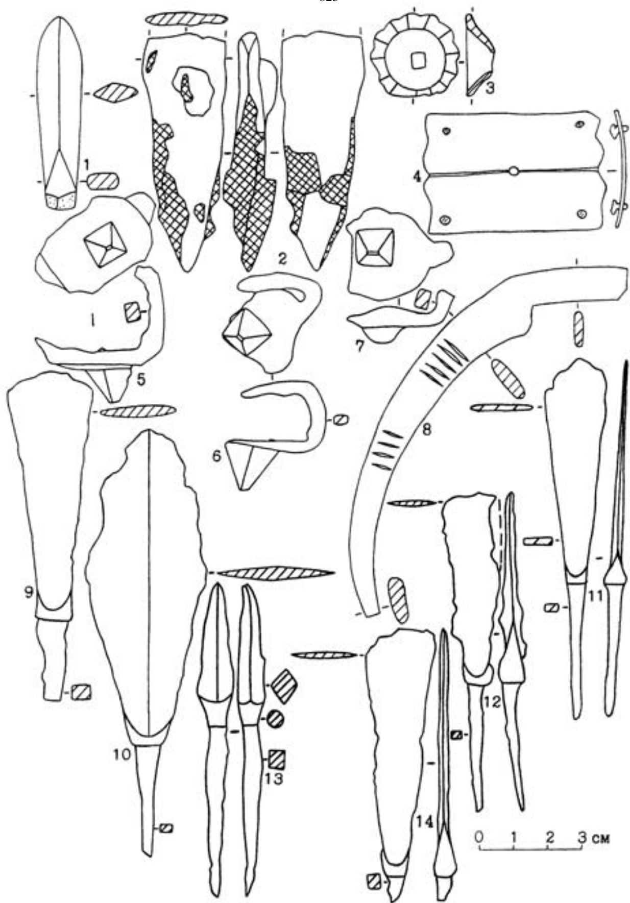
Рис.46. Наконечники стрел (1, 9-14), фрагмент кинжала (2), навершие шлема (3), панцирная пластина (4), ледоходные шипы (5-7), часть стремени
