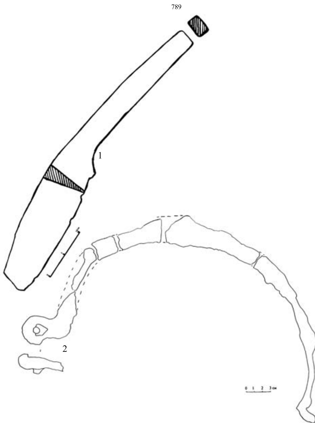
Рис.13. Железные чересло (1) и ручка ведра (2). 1 - Хмелевское I селище, подъемный материал 2001 г. 2 - селище Широкий Буерак, раскоп I-2001, яма 1.
