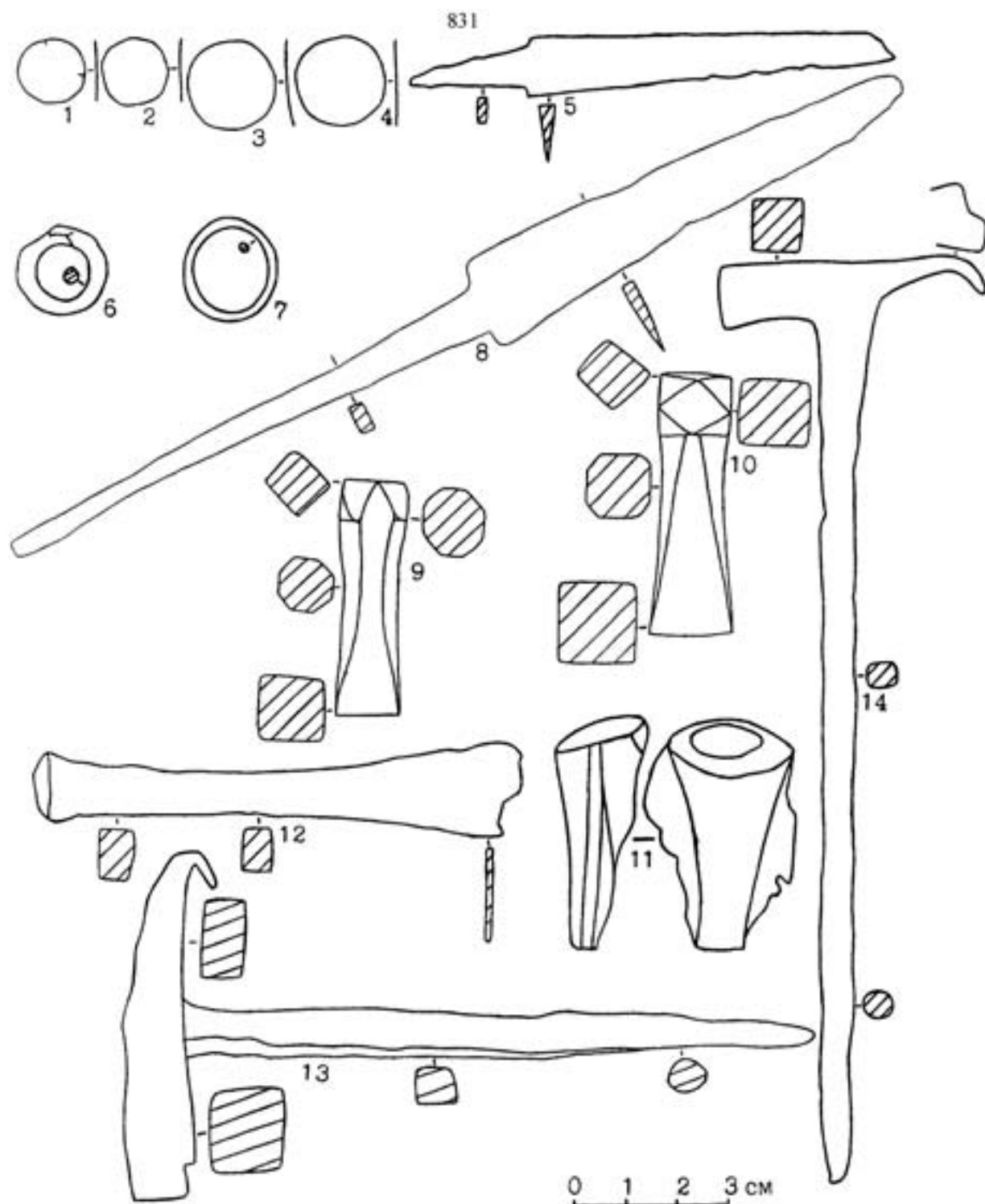
Рис.51. Пластинки (1-4), ножи (5, 8), кольца (6-7), наковаленки (9-10), заполнение литникового канала (11), зубило (12) и ювелирные молоточки (13-14). Увекское городище.
