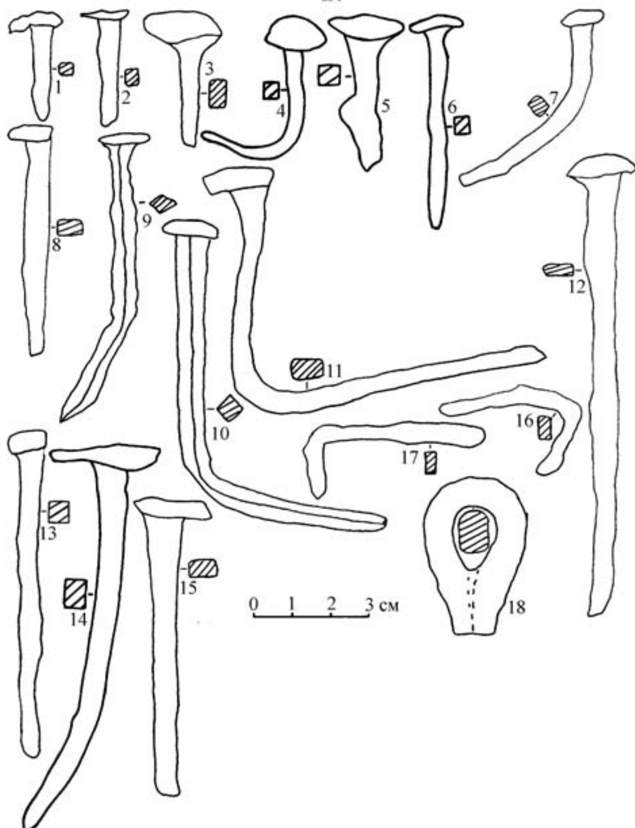
Рис.54. Железные гвозди (1-15), скобы (16-17) и пробой (18). 1-3,7-13,15-18 - Хмелевское I селище, раскоп II-2000, яма 1 (1-2,9), подъемный материал 2000-2001 гг. (3,7-8,10-13,15-18). 4-6,14 - Багаевское селище, раскоп I-2007, яма 4 (4-5), культурный слой (6,14).
