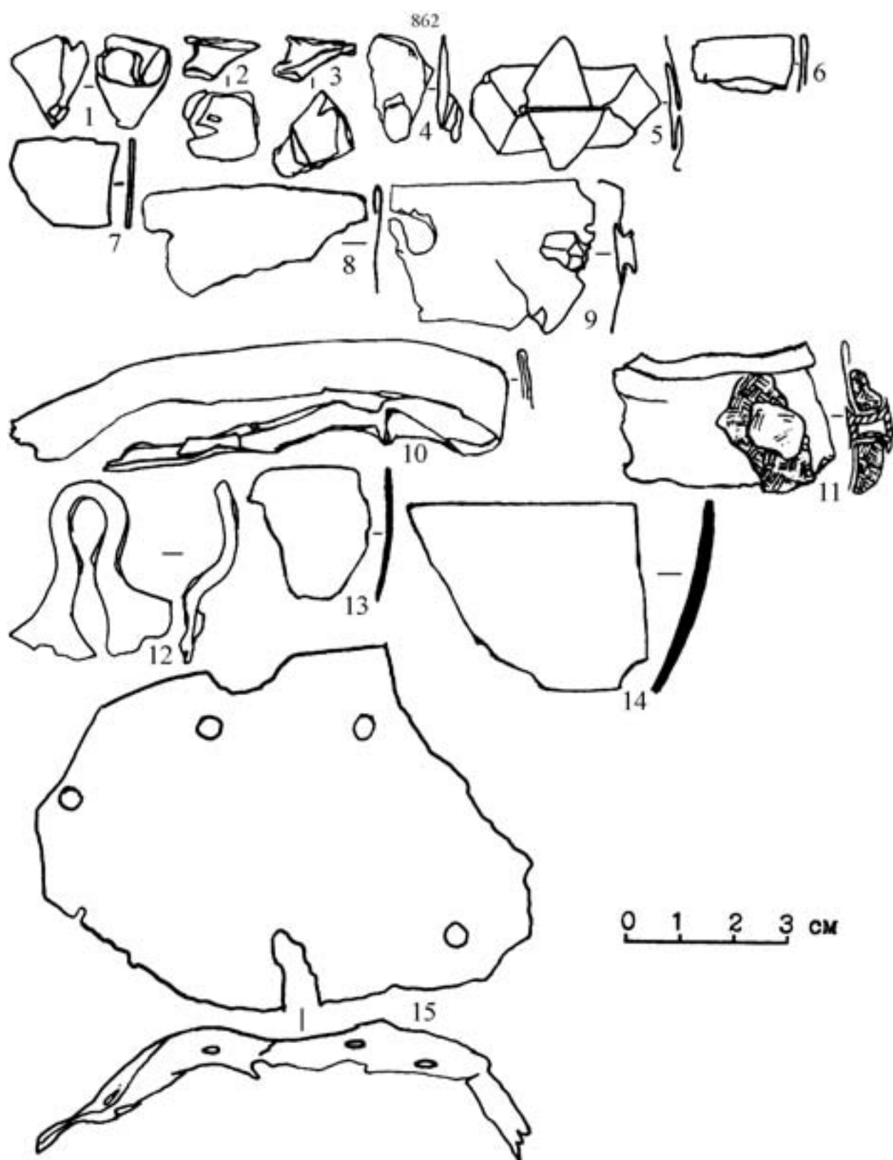
Рис.76. Бронзовые заклепки (1-5), ушко (12), фрагменты кованых (6-11) и литых (13-14) сосудов, оковка (15).
