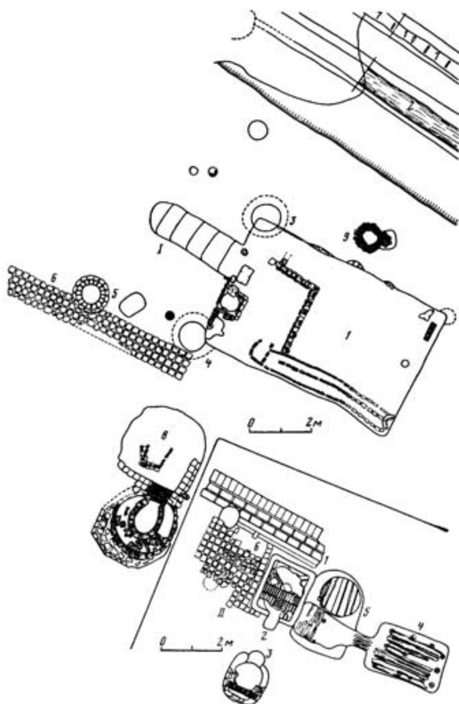
Рис.29. Детали планов раскопа II Селитренного городища с горнами 15 и 17-18, служившими для обжига неполивной керамики, и горнами 2-3 и 14 для обжига поливной посуды (по: Федоров-Давыдов Г.А., Булатов Н.М. Керамическая мастерская Селитренного городища // Сокровища сарматских вождей и древние города Поволжья. - М.: Наука, 1989. - С.138, рис.5). I – детали плана раскопа I, II (1970-1971): 1 – землянка 2, 2 – канава 1, 3 – горн 15, 4 – горн 17, 5 – колодец, 6 – стена усадьбы, 7 – канава 2, 8 – горн 14, 9 – горн 18; II – деталь плана раскопа II (1968): 1 – стена усадьбы, 2 – горн 3, 3 – горн 2, 4 – яма 22а, 5 – яма 22б, 6 – дом 1.
