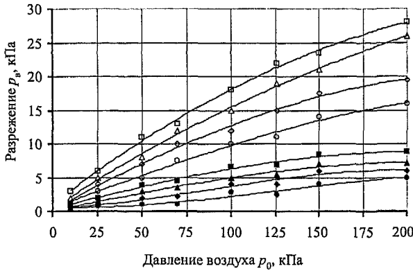
Рис. 2. Зависимость разрежения p_a в центральном отверстии от давления воздуха в устройстве p_0 : воздушный поток без закрутки – \square – h = 0,0006 м, K = 0,00696 м; – \blacktriangle – h = 0,00046 м, K = 0,0067 м; – \blacklozenge – h = 0,0004 м, K = 0,0064 м; – \circ – h = 0,003 м, K = 0,0062 м; воздушный поток вихревой – \blacksquare – h = 0,0006 м, K = 0,00696 м; – \blacktriangle – h = 0,00046 м, K = 0,0067 м; – \blacklozenge – h = 0,0004 м, K = 0,0064 м; – \bullet – h = 0,0003 м, K = 0,0062 м
