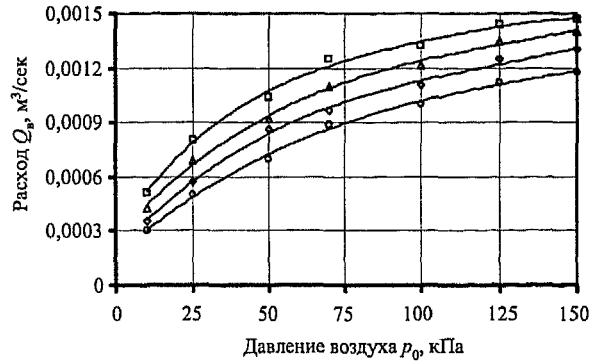
Рис. 3. Зависимость расхода Q_a в центральном отверстии от давления воздуха в устройстве p_0 : воздушный поток без закрутки – \square – h = 0,0006 м, K = 0,00696 м; – \triangle – h = 0,00046 м, K = 0,0067 м; – \diamond – h = 0,0004 м, K = 0,0064 м; – \circ – h = 0,003 м, K = 0,0062 м
