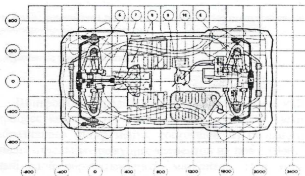
Рис. 3. Проекты городских автомобилей особо малого класса
