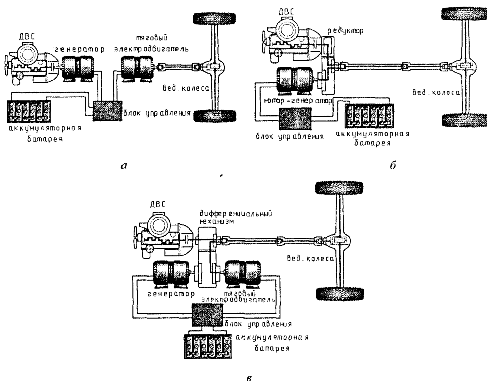
Рис. 2. Компонентные схемы силового привода с КЭУ:
