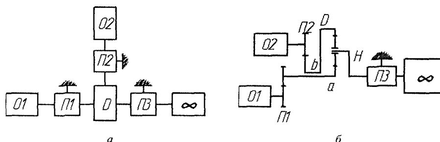
Рис. 3. Обобщенные схемы КЭУ параллельной схемы с планетарным дифференциальным согласующим редуктором: а – структурная; б – кинематическая
