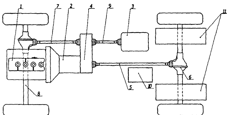
Рис. 4. Компоновочная схема силового привода полноприводного многоцелевого автомобиля с КЭУ параллельной схемы: 1 – ДВС; 2 – коробка передач; 3 – обратимая электрическая машина; 4 – раздаточная коробка; 5 – привод заднего моста; 6 – задний мост; 7 – привод переднего моста; 8 – передний мост; 9 – привод обратимой электрической машины; 10 – система управления тяговым электрооборудованием; 11 – электрические накопители энергии
