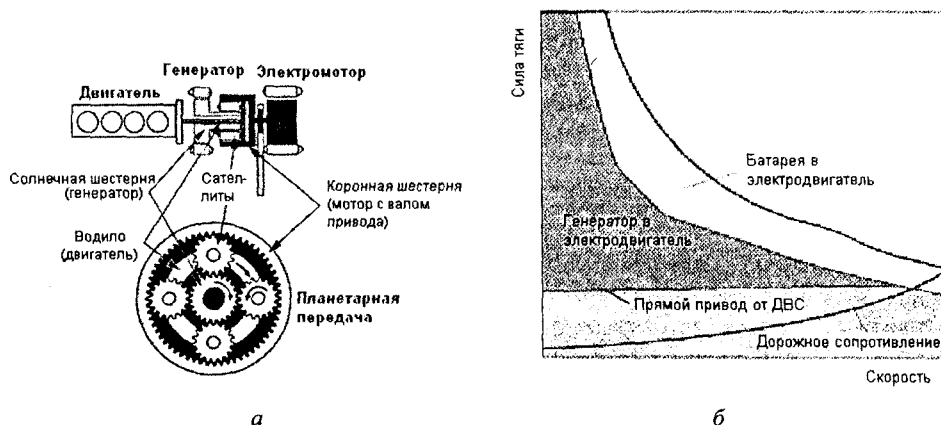
Рис. 5. КЭУ параллельно-последовательной схемы THS II: а – структурная схема; б – тяговая характеристика
