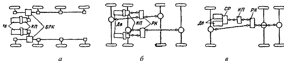
Рис. 1. Двухдвигательный силовой привод: а – бортовая схема; б – мостовая схема; в – с суммирующим редуктором
