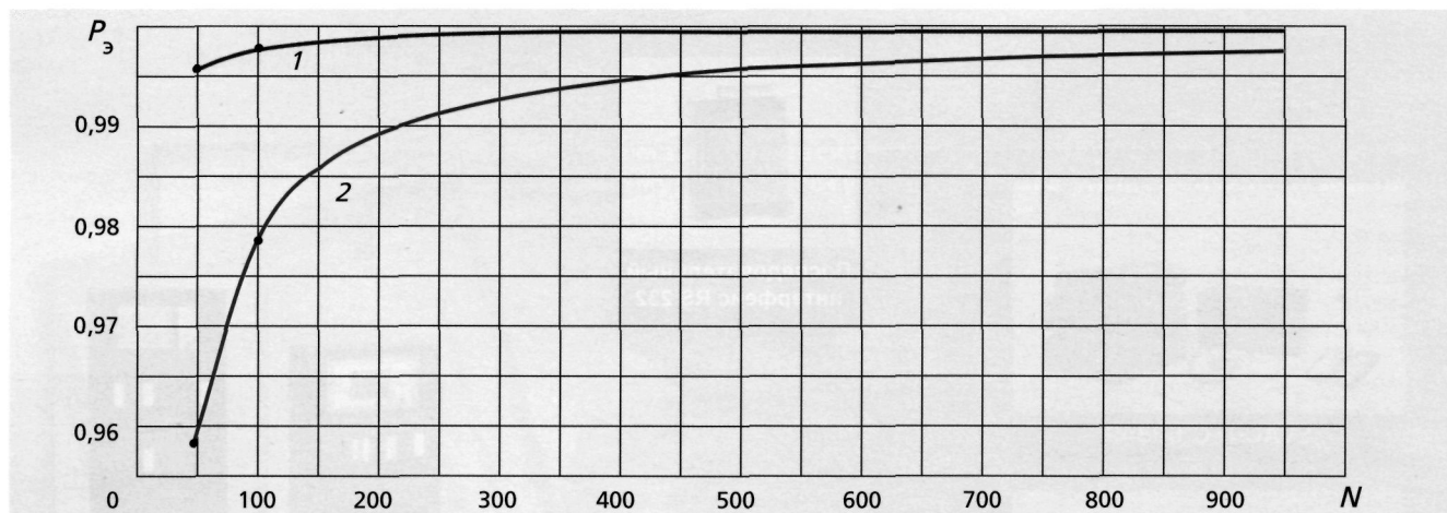
Рис. 1. Зависимость граничного значения вероятности эвакуации людей ( P_{э}^* ) от их числа ( N ) в здании образовательного учреждения при отсутствии (1) или наличии (2) в нем системы автоматического пожаротушения
