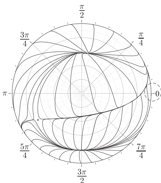
Рис. 18. Траектории движения треноги, в основании которой лежит треугольник, вытянутый вдоль оси симметрии ( h = 1, \mu = 1, \text{tg } \alpha = 0.05 ). Выделенная пунктиром область \tau -устойчивого поступательного движения вблизи ( \varphi = 0, \psi = 0 ) подробно исследована в параграфе 4.2 (рис. 8, рис. 9).
