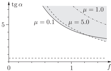
Рис. 10. Области \tau -устойчивого поступательного движения треноги при \mu = 0.1, 1.0, 5.0 и фиксированных R_2 = 1, h = 0.1 (выделены серым цветом над соответствующими кривыми).
