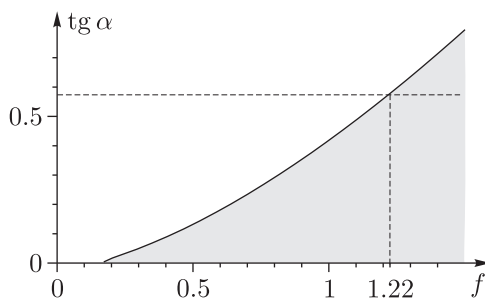
Рис. 3. Область \tau -устойчивого поступательного движения треугольной пайбы с параметрами h = 0.1, R_2 = 1, m = 1 (обозначена серым цветом). Горизонтальная пунктирная линия соответствует пайбе, опирающейся на плоскость равносторонним треугольным основанием ( \text{tg}\alpha = 1/\sqrt{3} ).
