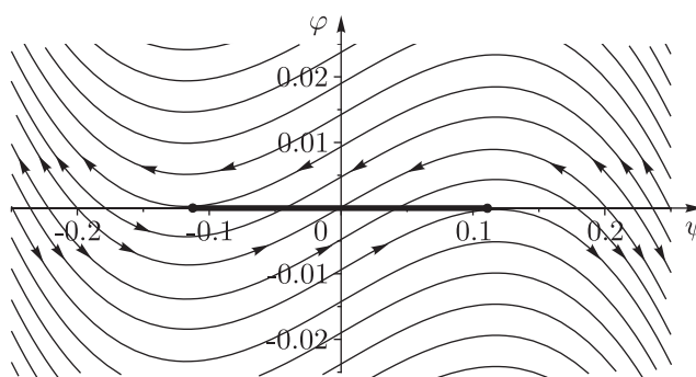
Рис. 5. Фазовый портрет и область \tau -устойчивого поступательного движения треугольной пайбы ( h = 0.1, R_2 = 1, m = 1, f = 0.5, \text{tg}\alpha = 0.1, g = 10 )
