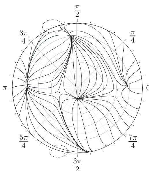
Рис. 19. Траектории движения треноги, в основании которой лежит треугольник, сплюснутый вдоль оси симметрии ( h = 1, \mu = 1, \text{tg } \alpha = 5 ). Выделенные пунктиром области \tau -устойчивого поступательного движения подробно исследованы в параграфе 4.2 (рис. 11, рис. 12).
