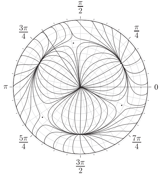
Рис. 16. Траектории движения треноги, в основании которой лежит равносторонний треугольник ( h = 1 , \mu = 1 ).
