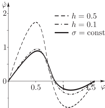
Рис. 13. Графики функции p(\varphi) при h = 0.1, 0.5 при фиксированных M = 1, f = 1, R = 1 .
