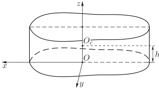
Рис. 1. Шайба на плоскости.
