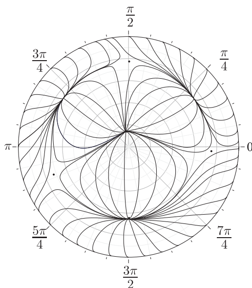
Рис. 17. Траектории движения треноги, в основании которой лежит равносторонний треугольник с неравномерным распределением масс в его вершинах ( h = 1, \mu = 1.5 ).
