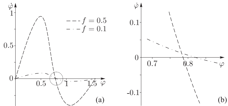
Рис. 14. (а) Графики функции p(\varphi) при f = 0.1, 0.5 при фиксированных M = 1, h = 1, R = 1 . (б) Увеличенная область пересечения p(\varphi) с осью абсцисс.
