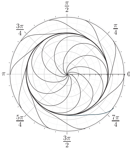
Рис. 15. Траектории движения редуцированной системы круглой однородной шайбы при R = 1 , M = 1 , h = 0.1 , f = 0.5 .
