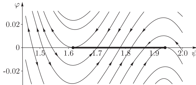
Рис. 12. Фазовый портрет вблизи области \tau -устойчивого поступательного движения треноги \varphi = 0, 1.615 < \psi < 1.935 при фиксированных h = 0.1, R_2 = 1, \mu = 1, f = 3, \text{tg } \alpha = 5, g = 10 .
