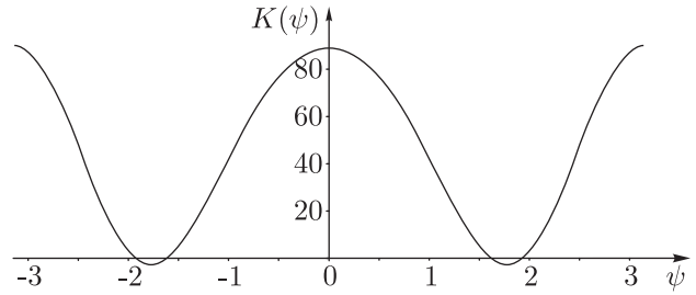
Рис. 11. График функции K(\psi) треноги ( h = 0.1, R_2 = 1, \mu = 1, f = 3, \text{tg } \alpha = 5 ). При выполнении условия K(\psi) < 0 поступательное движение \tau -устойчиво.
