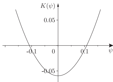
Рис. 4. График функции K(\psi) треугольной пайбы ( h = 0.1, R_2 = 1, m = 1, f = 0.5, \text{tg}\alpha = 0.1, g = 10 ). При K(\psi) < 0 поступательное движение \tau -устойчиво.
